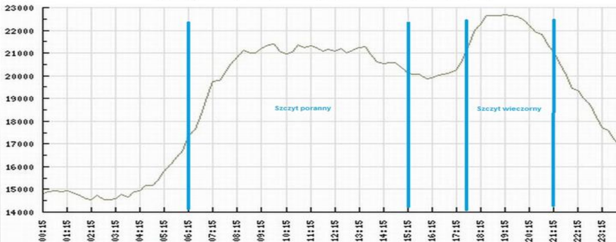
Typowy przebieg szczytów mocy systemu energetycznego [MW]
